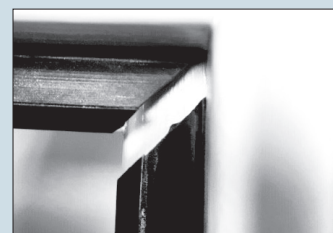
Dichtungsmontage Rahmenstock: falsch ✗
